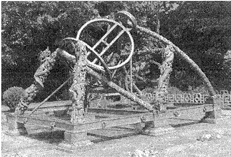
南京紫禁山天文台の簡儀(天文観測器)
